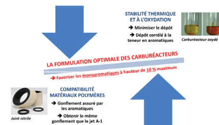
Optimisation de la formulation d'un carburéacteur.
