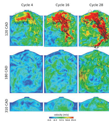
Champs de vitesses instantanées résolues en LES à trois angles vilebrequin, et pour trois cycles du transitoire : cycle 4 (1 000 tr/min), cycle 16 (1 400 tr/min) et cycle 28 (1 800 tr/min).
