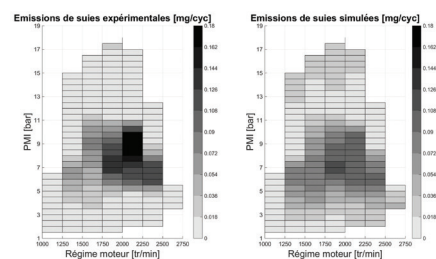
Comparaison des quantités de suies mesurées et calculées dans le domaine de fonctionnement du moteur b .
