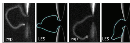
Fig. 1 - Comparaison expérience vs LES pour deux visualisations de l'arc électrique.
